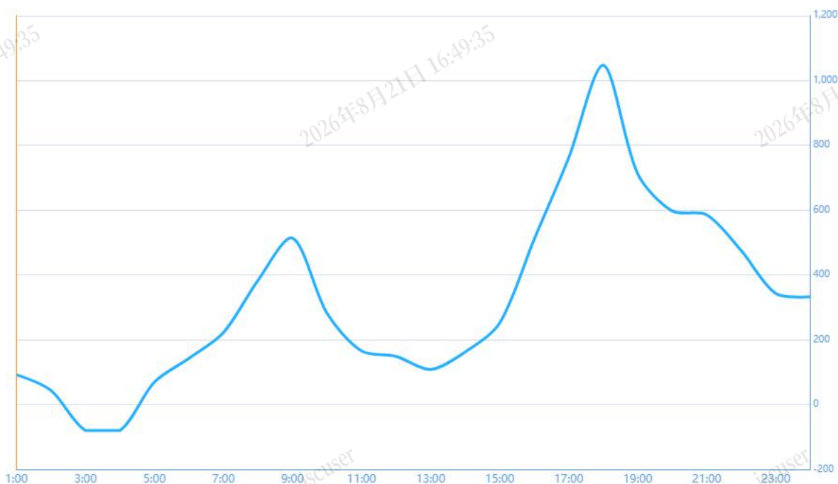
图 2 1 月 13 日日前市场用电侧价格
