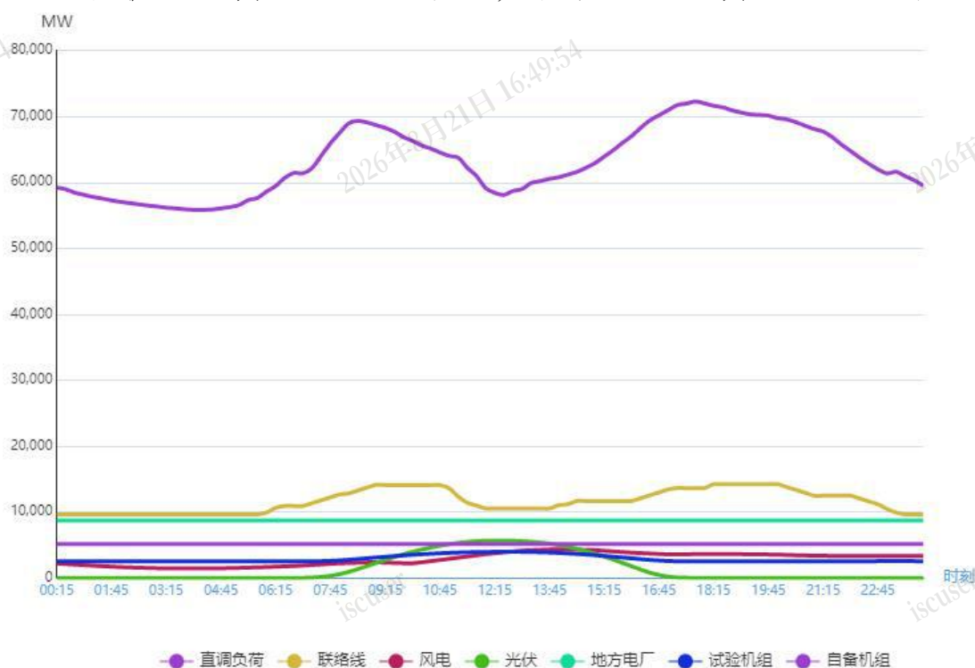
图 1 1 月 17 日负荷及电源出力预测情况
