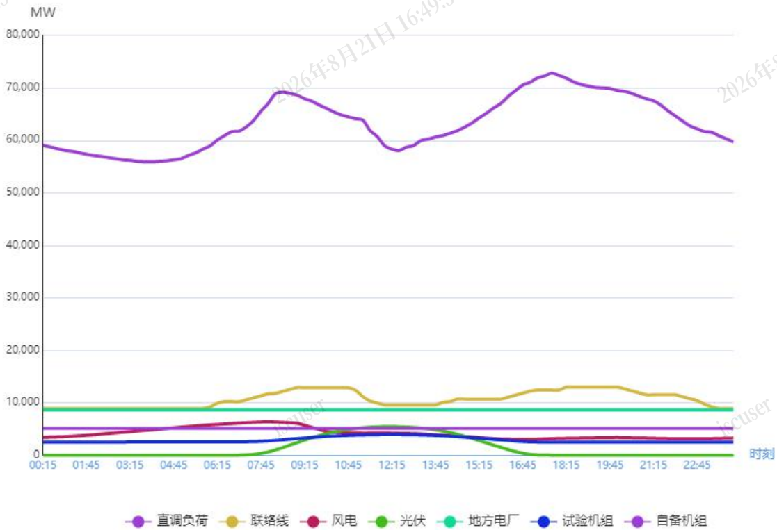
图1 1月18日负荷及电源出力预测情况
