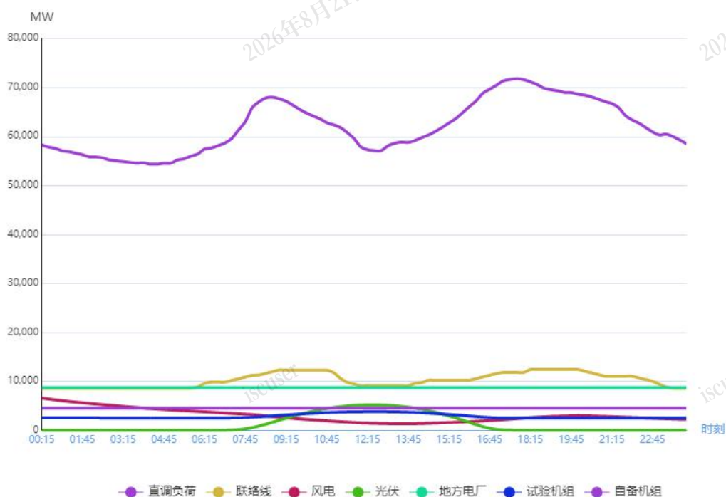
图 1 1月20日负荷及电源出力预测情况
