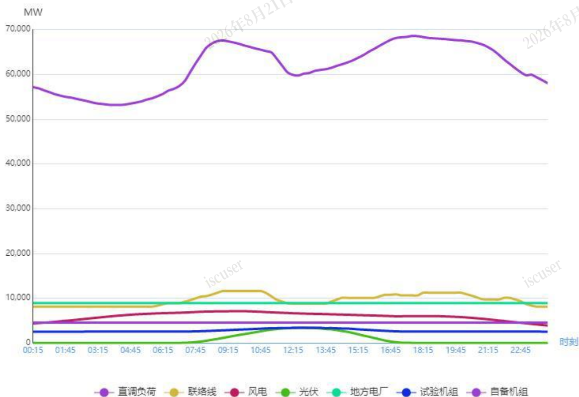
图 1 1 月 23 日负荷及电源出力预测情况
