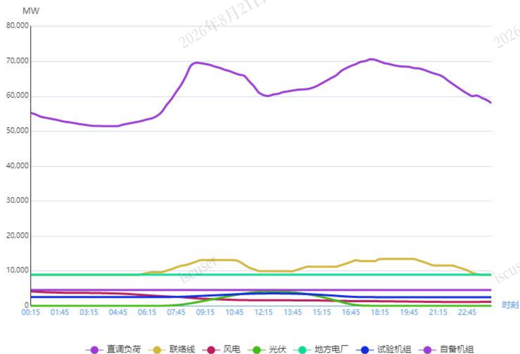
图 1 1 月 24 日负荷及电源出力预测情况
