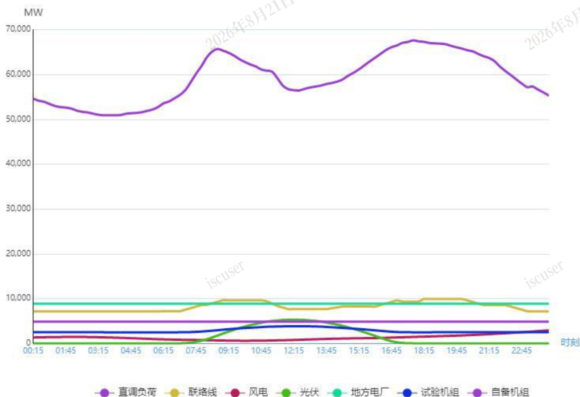
图 1 1 月 25 日负荷及电源出力预测情况
