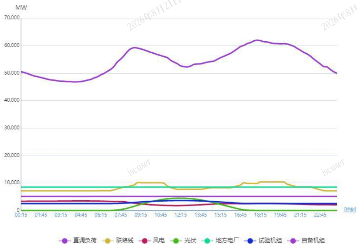
图 1 1 月 27 日负荷及电源出力预测情况
