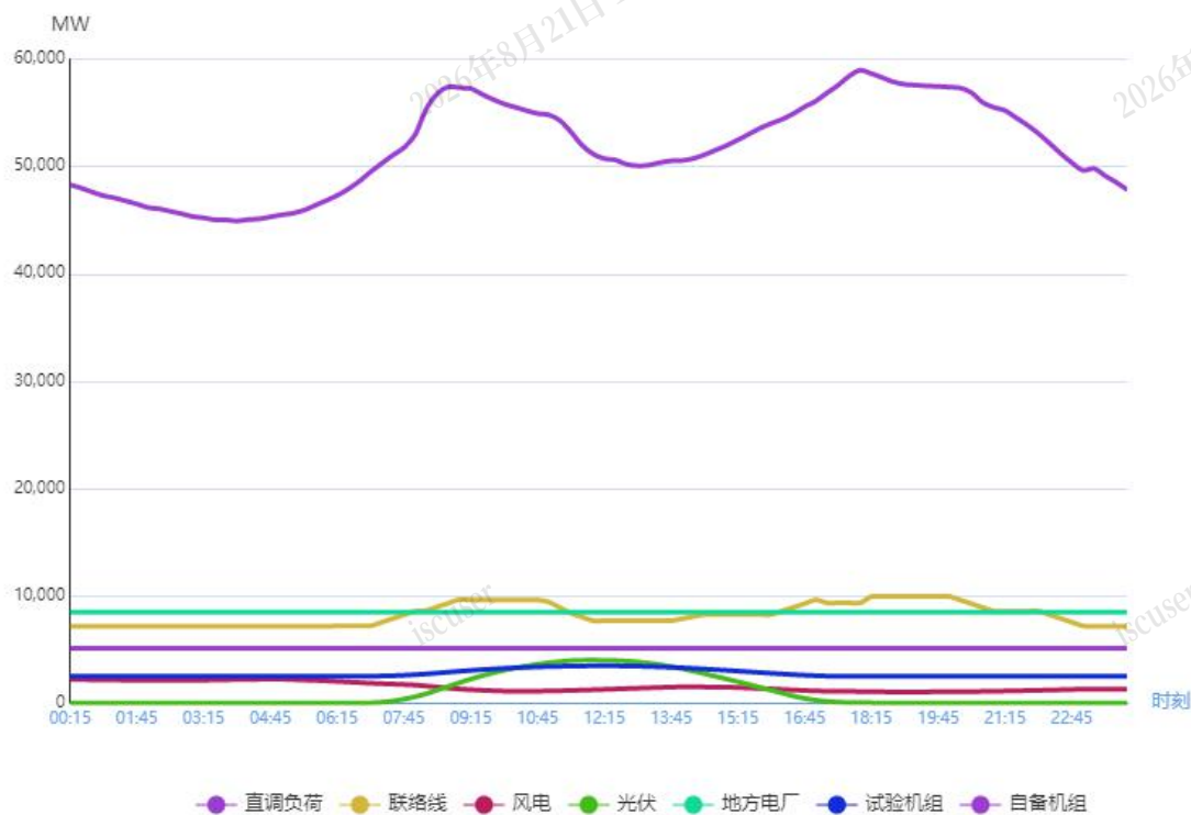
图 1 1 月 28 日负荷及电源出力预测情况
