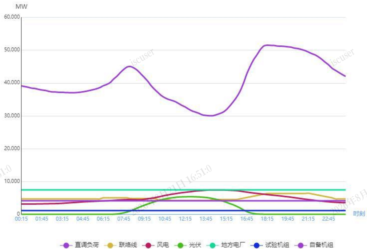
图 1 2月4日负荷及电源出力预测情况
