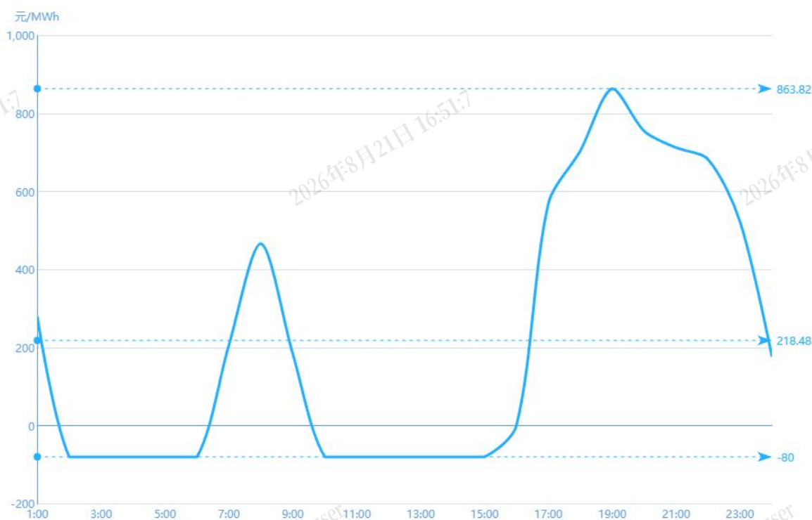
图 3 2 月 5 日实时市场用电侧价格
