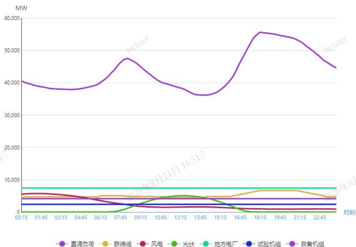
图 1 2月6日负荷及电源出力预测情况
