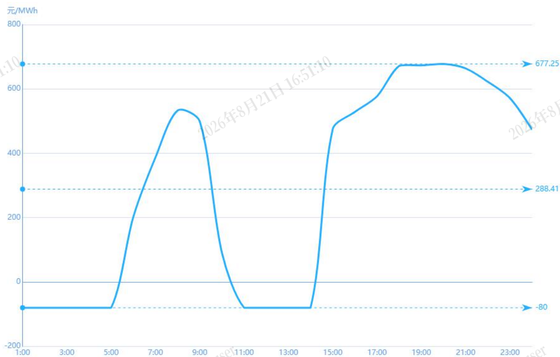
图 3 2 月 6 日实时市场用电侧价格
