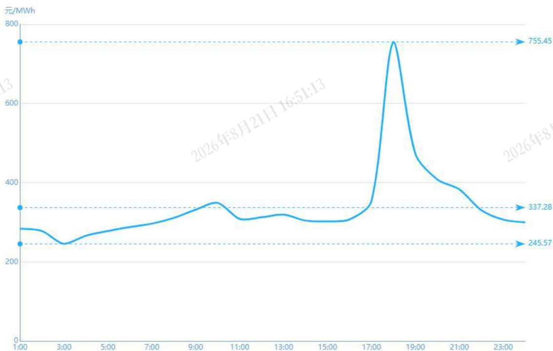
图 4 2 月 7 日实时市场用电侧价格
