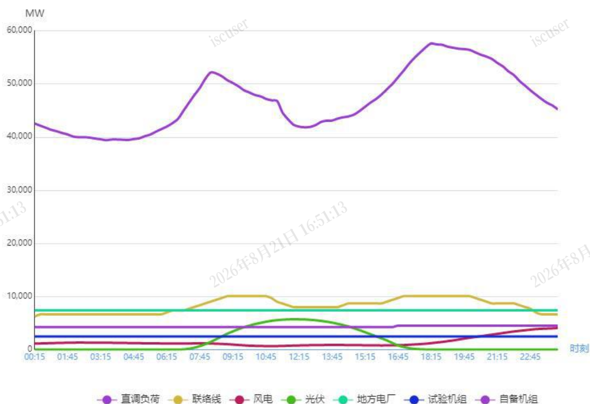
图2 2月8日负荷及电源出力预测情况
