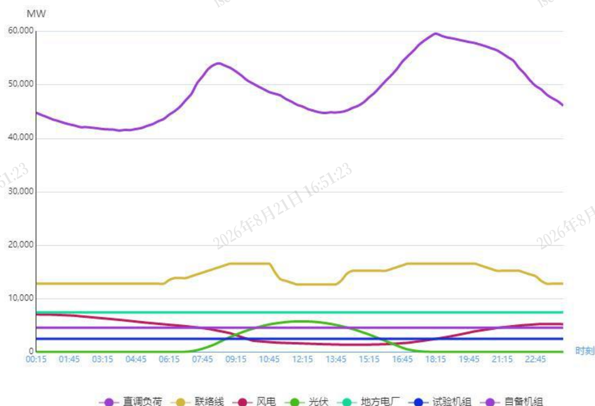
图1 2月10日负荷及电源出力预测情况
