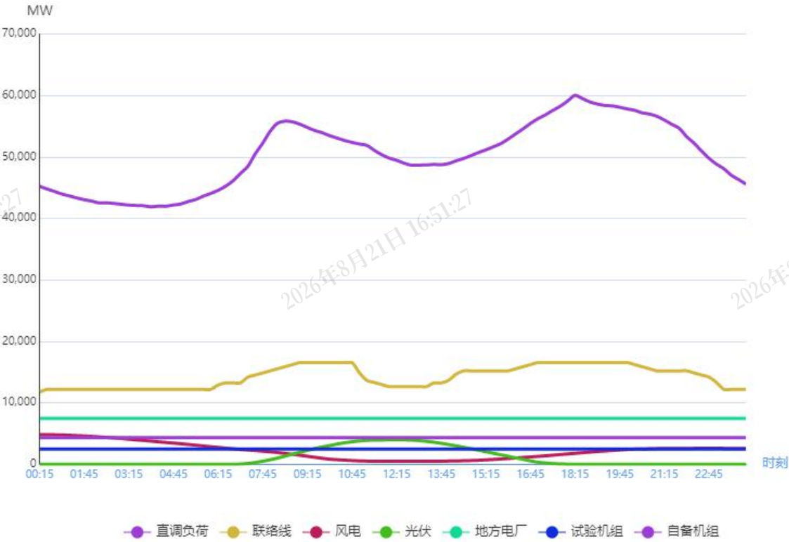
图 1 2月11日负荷及电源出力预测情况
