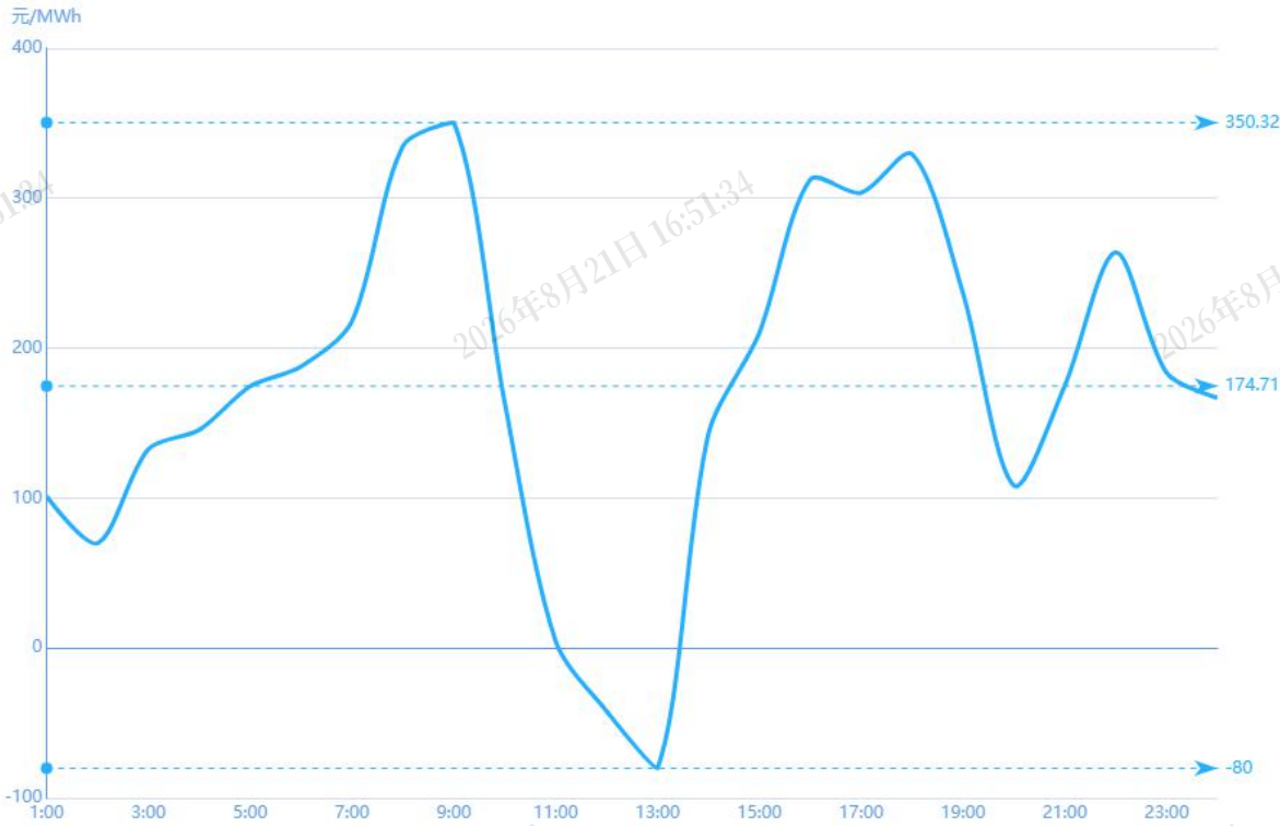
图 4 2 月 12 日实时市场用电侧价格
