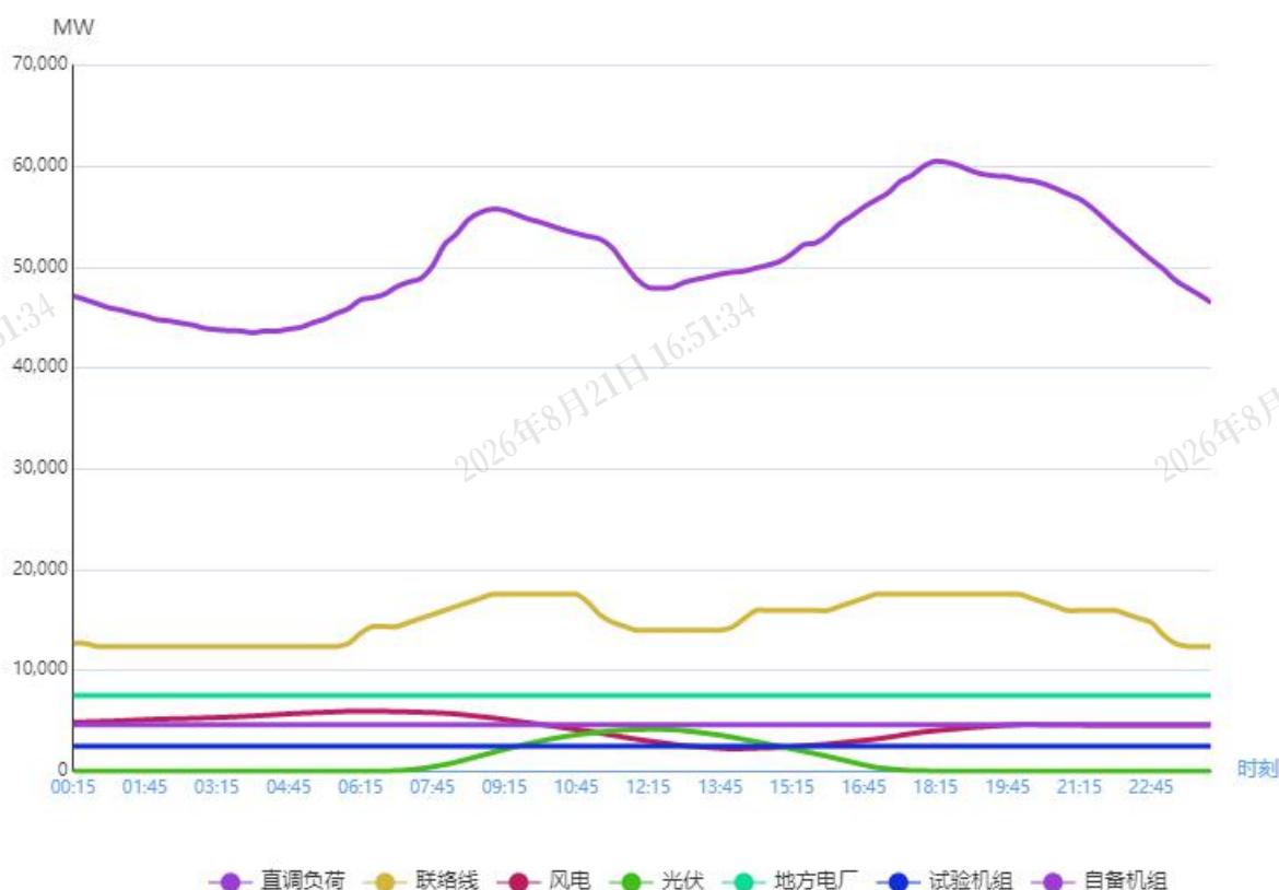
图 2 2月13日负荷及电源出力预测情况
