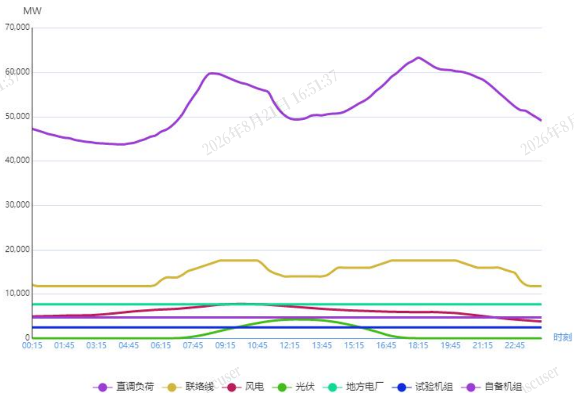
图1 2月14日负荷及电源出力预测情况
