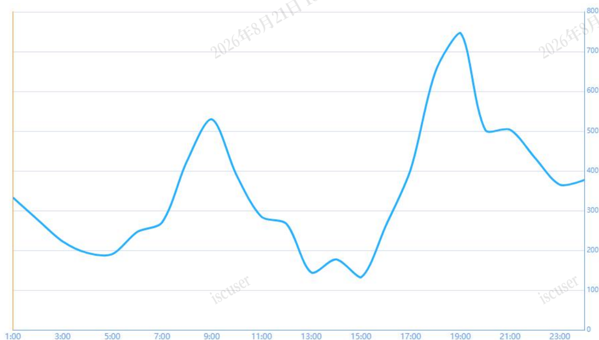
图 2 2 月 16 日日前市场用电侧价格
