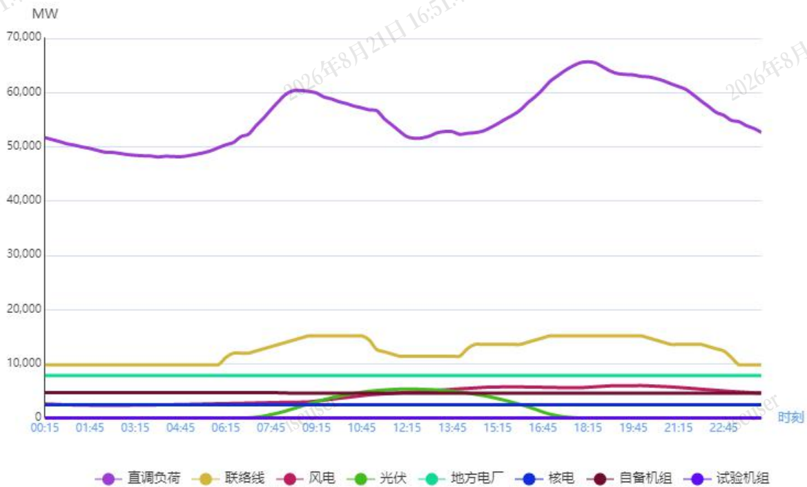
图1 2月16日负荷及电源出力预测情况
