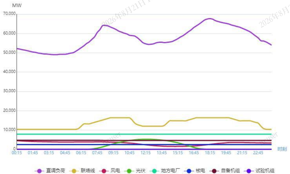
图1 2月17日负荷及电源出力预测情况
