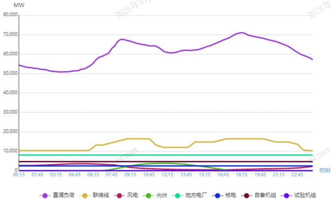
图1 2月18日负荷及电源出力预测情况
