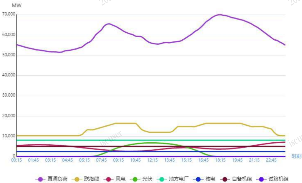
图 1 2月20日负荷及电源出力预测情况
