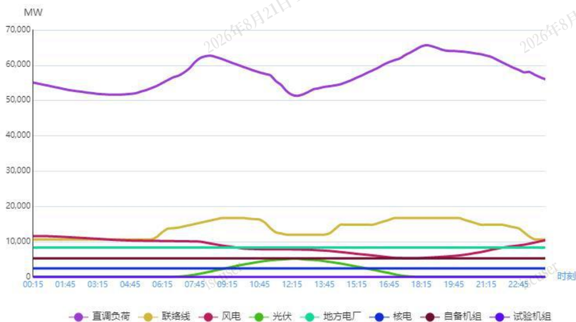
图 1 2 月 28 日负荷及电源出力预测情况
