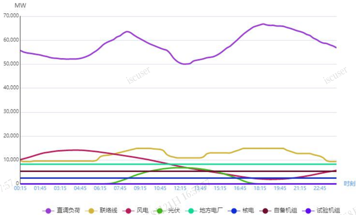
图 1 3 月 1 日负荷及电源出力预测情况
