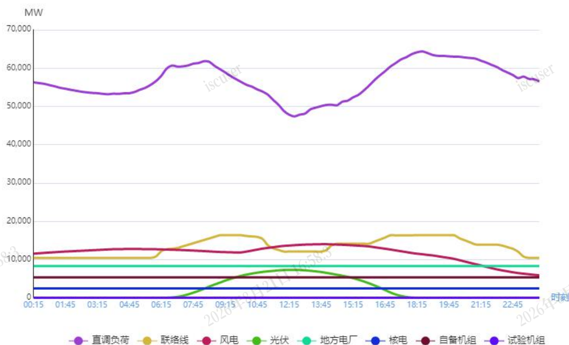
图1 3月3日负荷及电源出力预测情况
