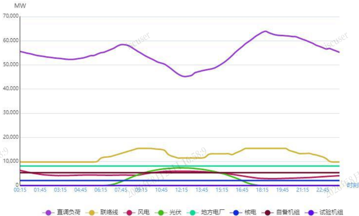
图1 3月5日负荷及电源出力预测情况
