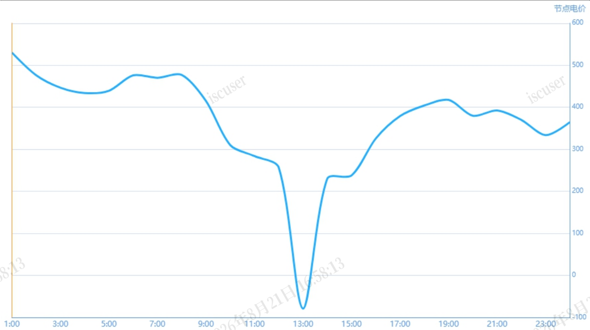
图2 3月6日日前市场用电侧价格
