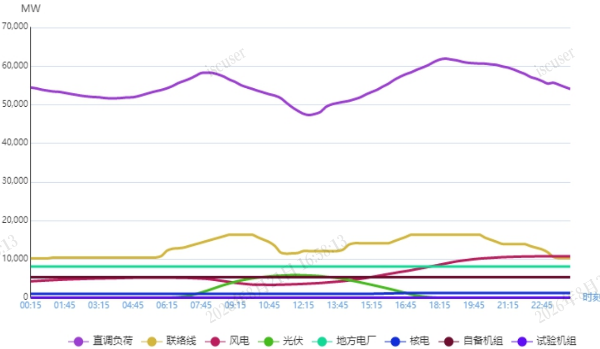
图 1 3月6日负荷及电源出力预测情况
