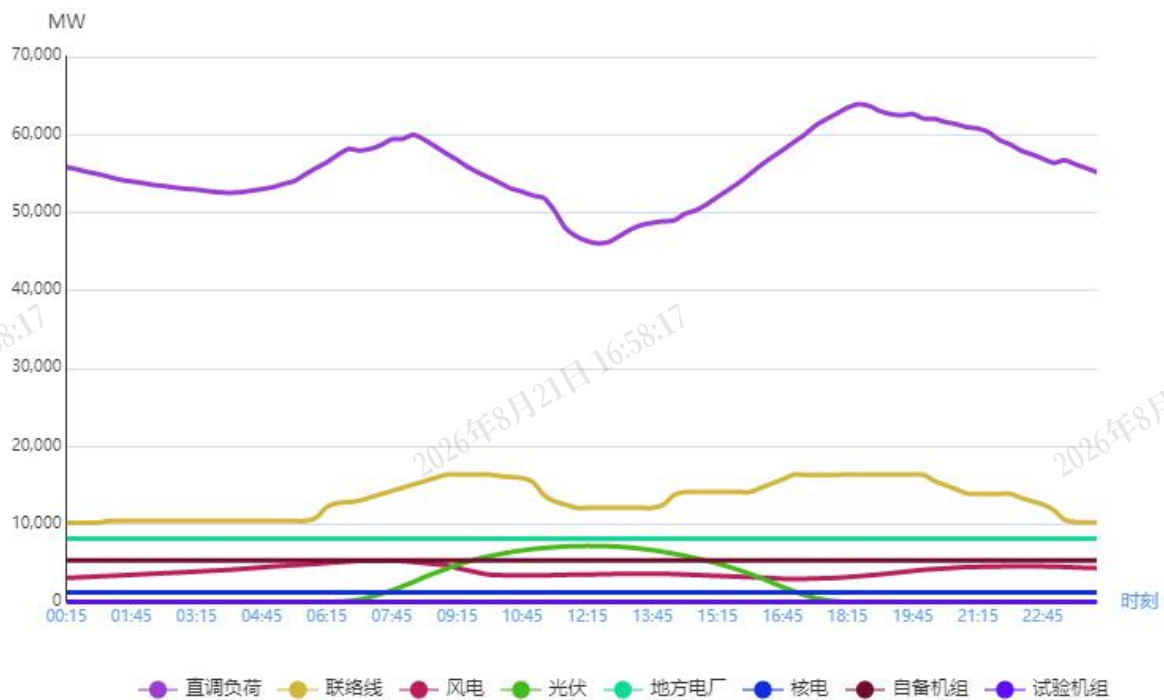
图1 3月7日负荷及电源出力预测情况
