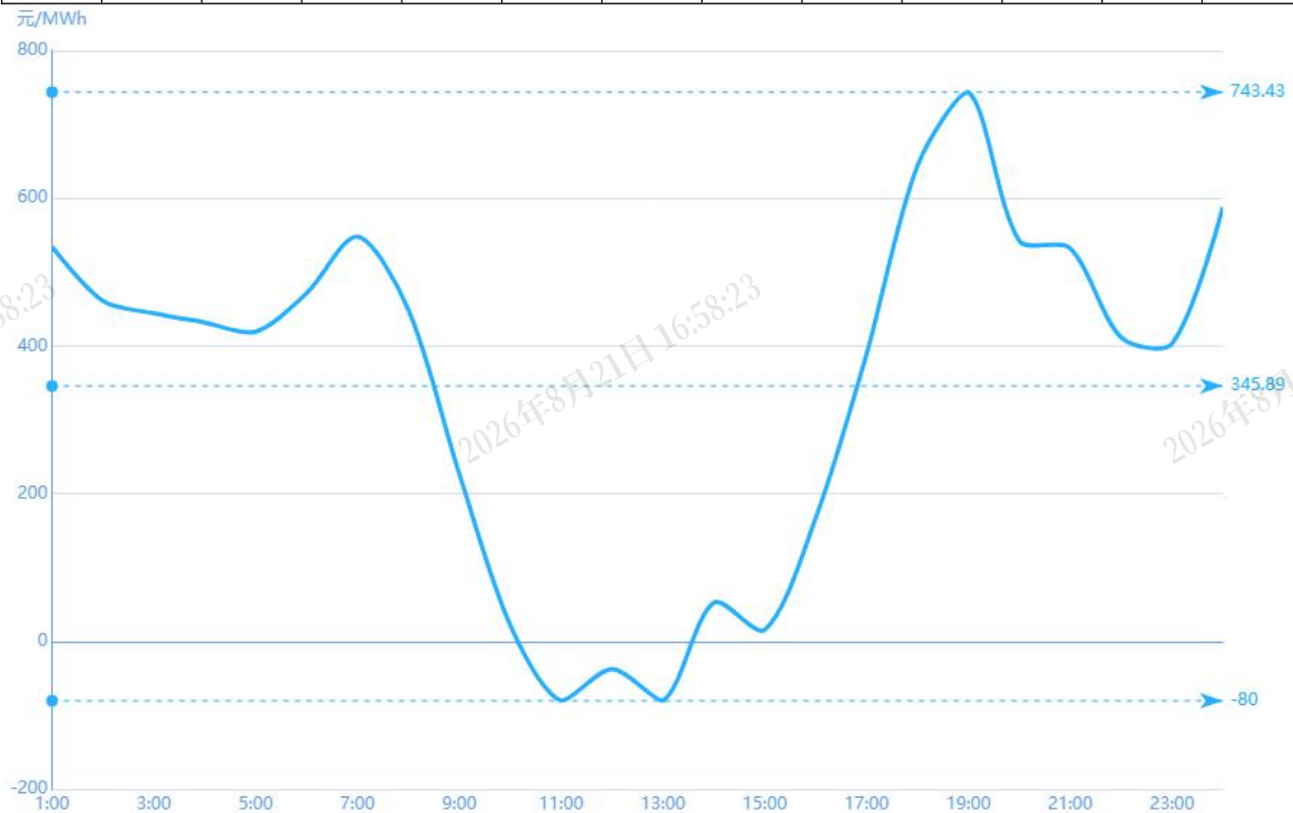
图 3 3月8日实时市场用电侧价格
