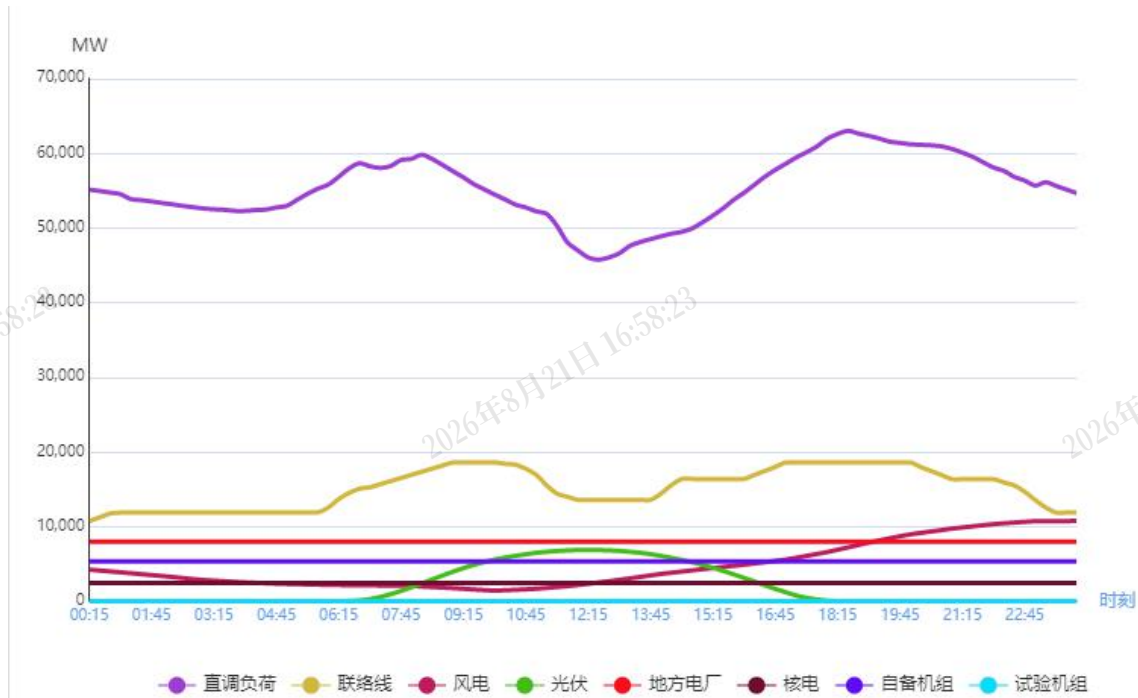
图1 3月9日负荷及电源出力预测情况
