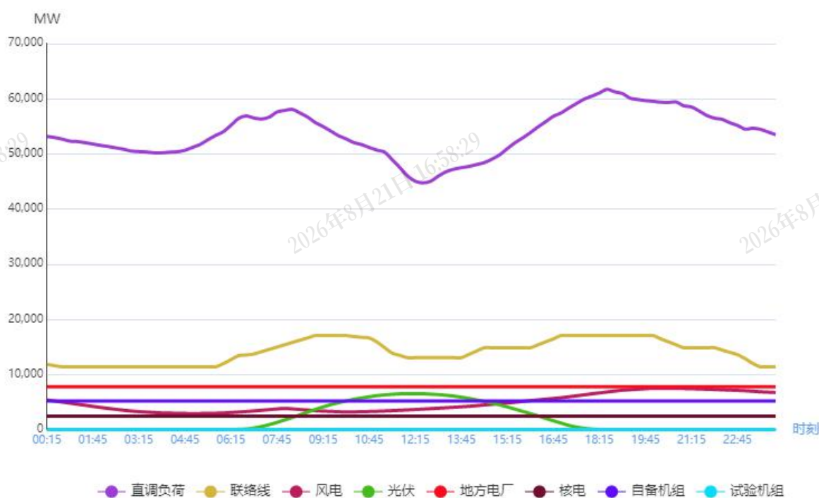
图1 3月11日负荷及电源出力预测情况
