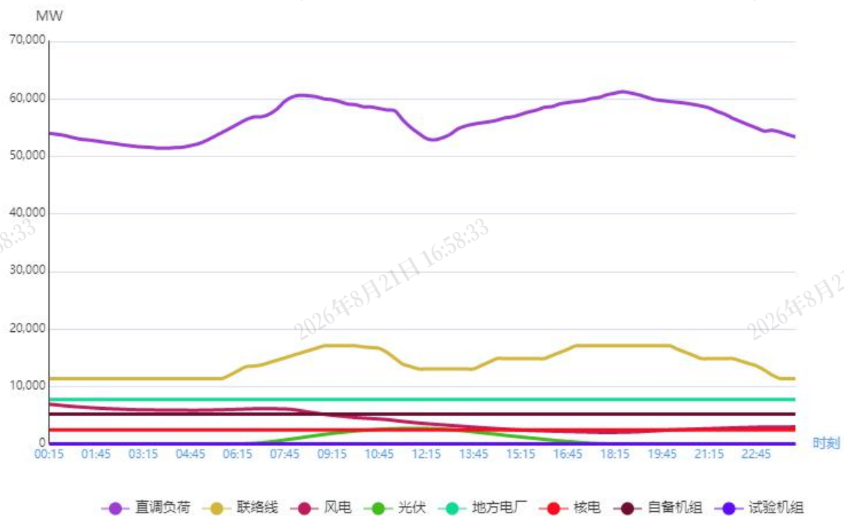
图2 3月12日负荷及电源出力预测情况
