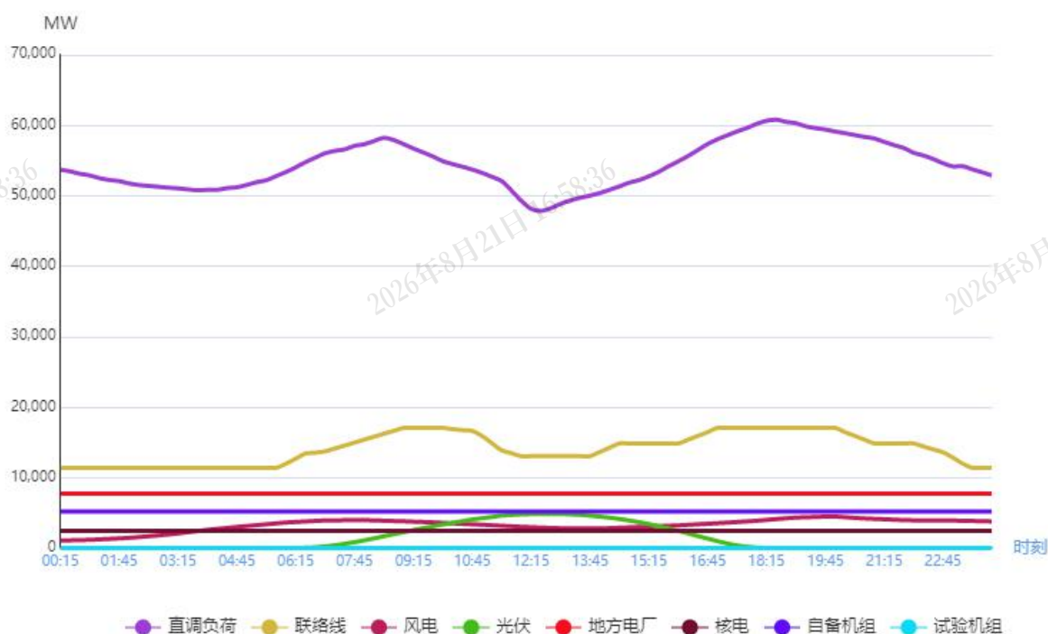
图2 3月13日负荷及电源出力预测情况
