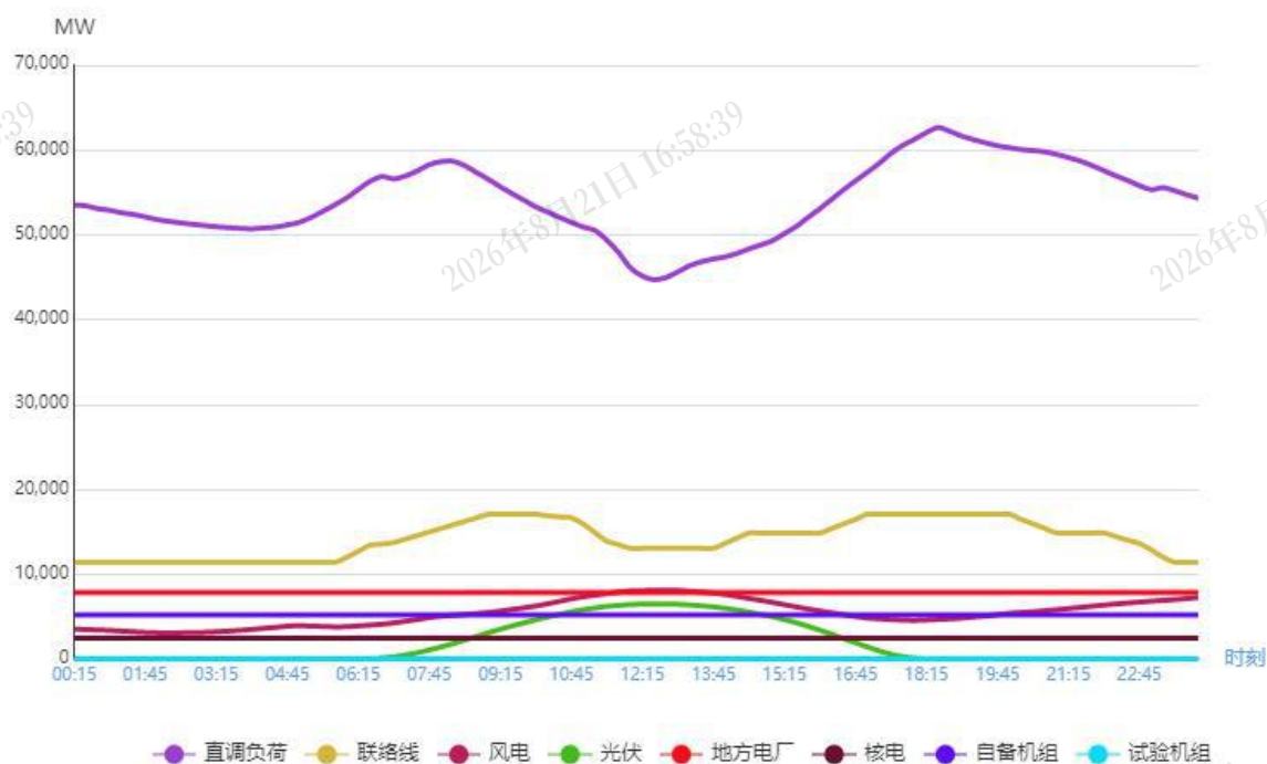
图1 3月14日负荷及电源出力预测情况
