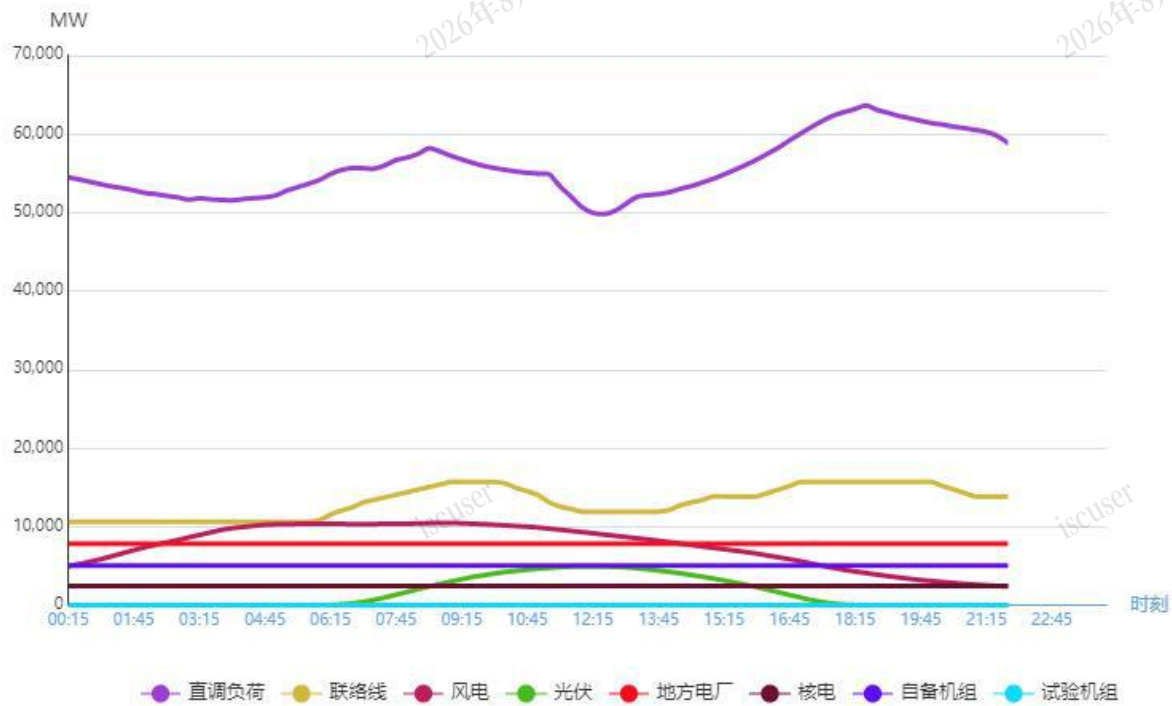
图1 3月19日负荷及电源出力预测情况
