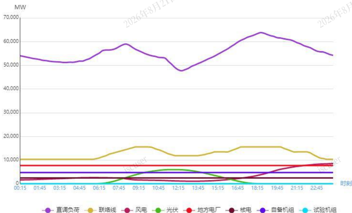
图 1 3 月 22 日负荷及电源出力预测情况
