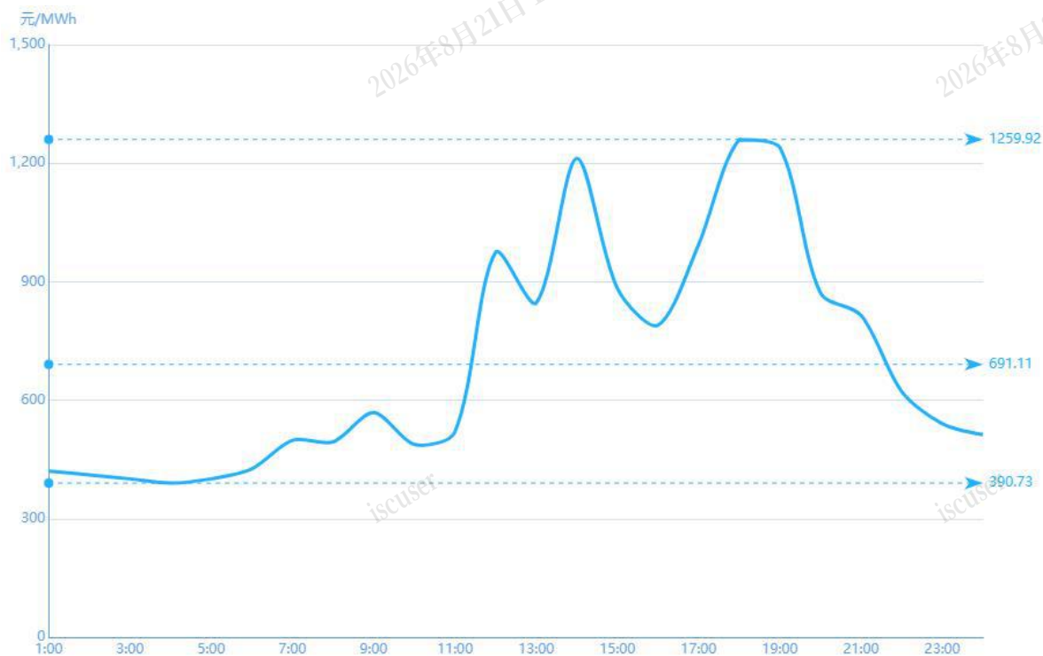
图3 3月21日实时市场用电侧价格
