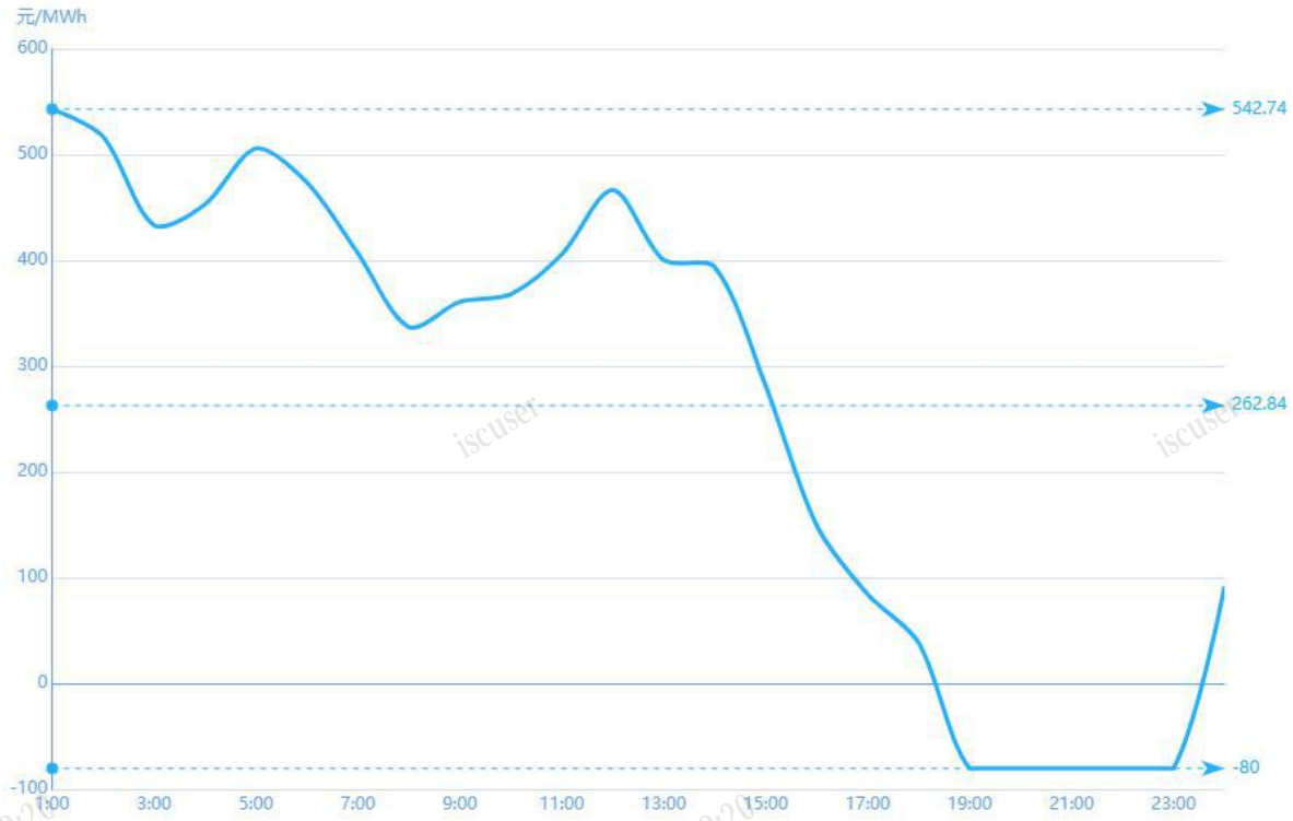
图3 3月25日实时市场用电侧价格
