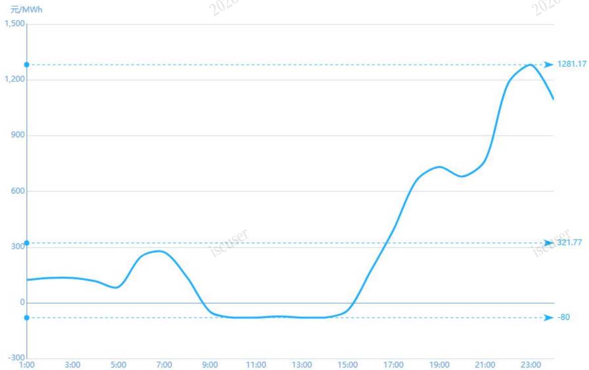
图3 3月29日实时市场用电侧价格
