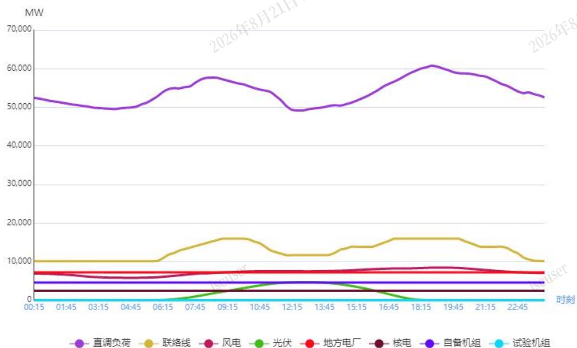
图 1 3 月 30 日负荷及电源出力预测情况
