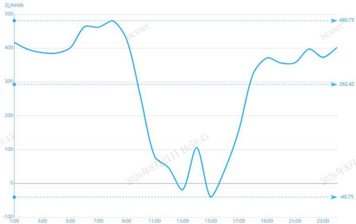
图3 3月31日实时市场用电侧价格
