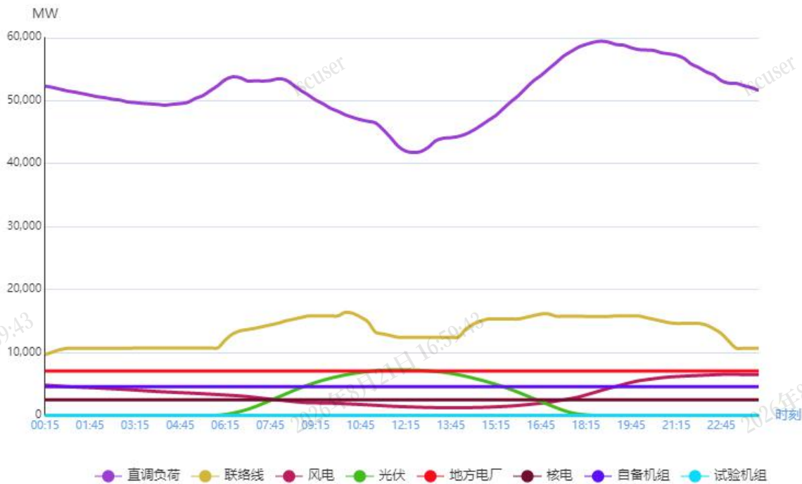
图 1 4月1日负荷及电源出力预测情况
