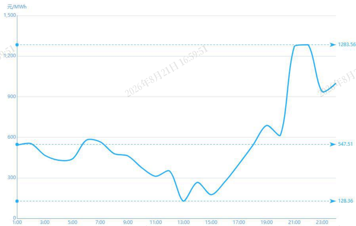
图 3 4 月 2 日实时市场用电侧价格
