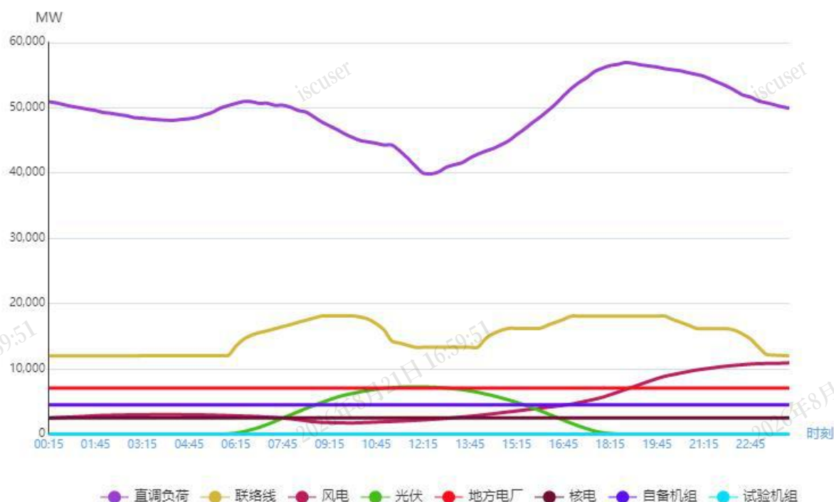
图1 4月3日负荷及电源出力预测情况
