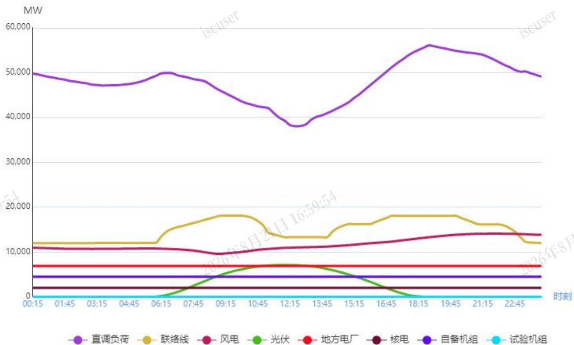
图1 4月4日负荷及电源出力预测情况
