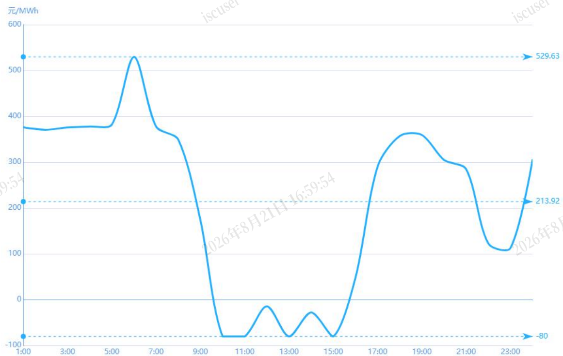
图3 4月3日实时市场用电侧价格
