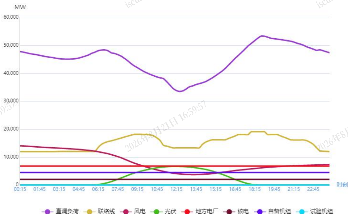
图2 4月5日负荷及电源出力预测情况
