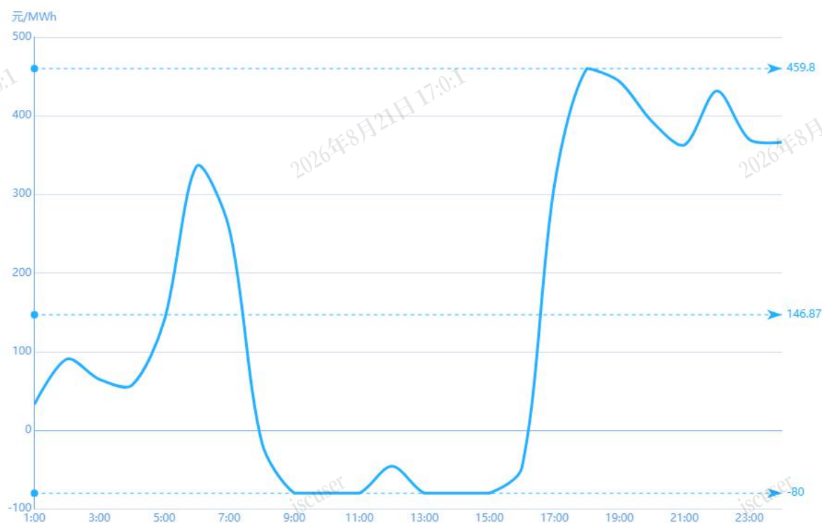
图 3 4 月 5 日实时市场用电侧价格
