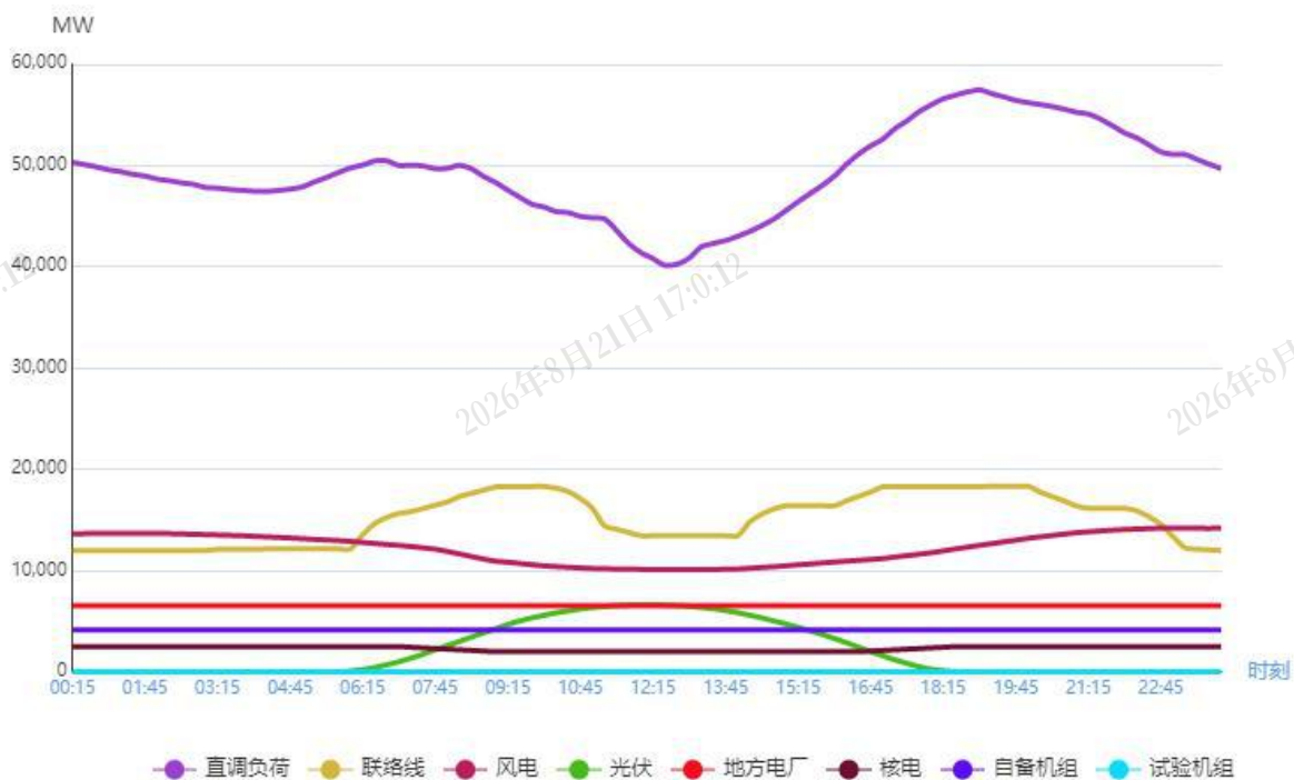
图1 4月9日负荷及电源出力预测情况
