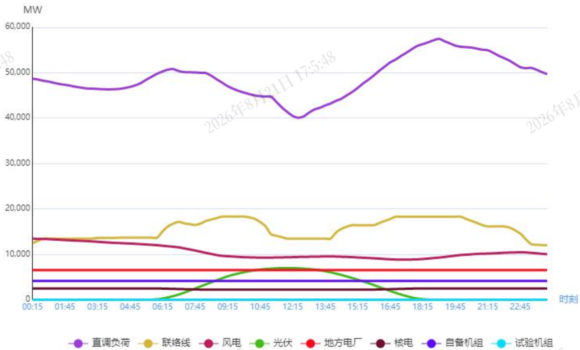
图1 4月11日负荷及电源出力预测情况
