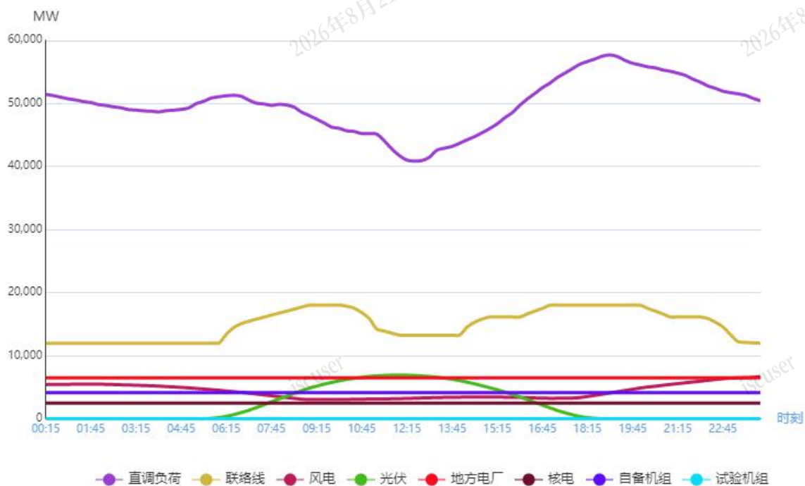
图1 4月16日负荷及电源出力预测情况
