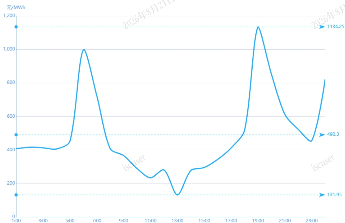
图3 4月18日实时市场用电侧价格
