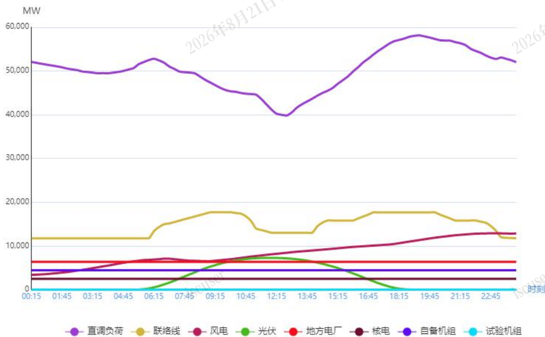
图 1 4 月 23 日负荷及电源出力预测情况
