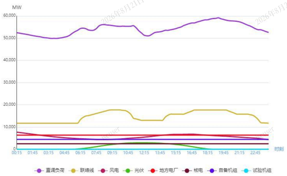
图 1 4 月 25 日负荷及电源出力预测情况
