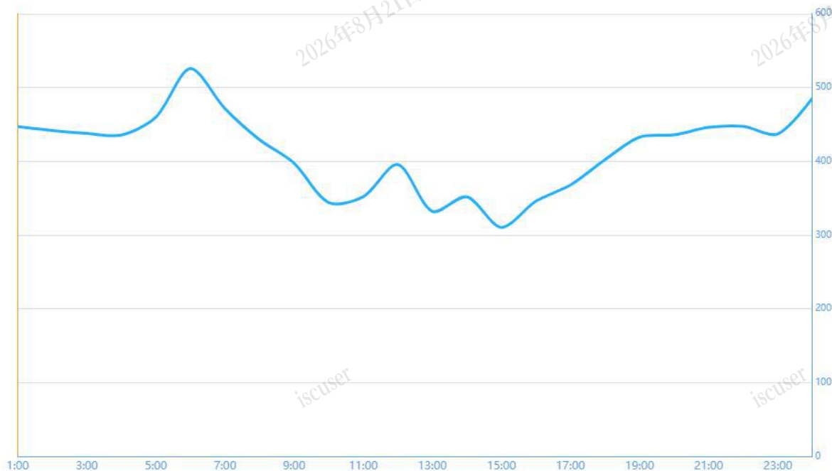
图 2 4 月 25 日日前市场用电侧价格
