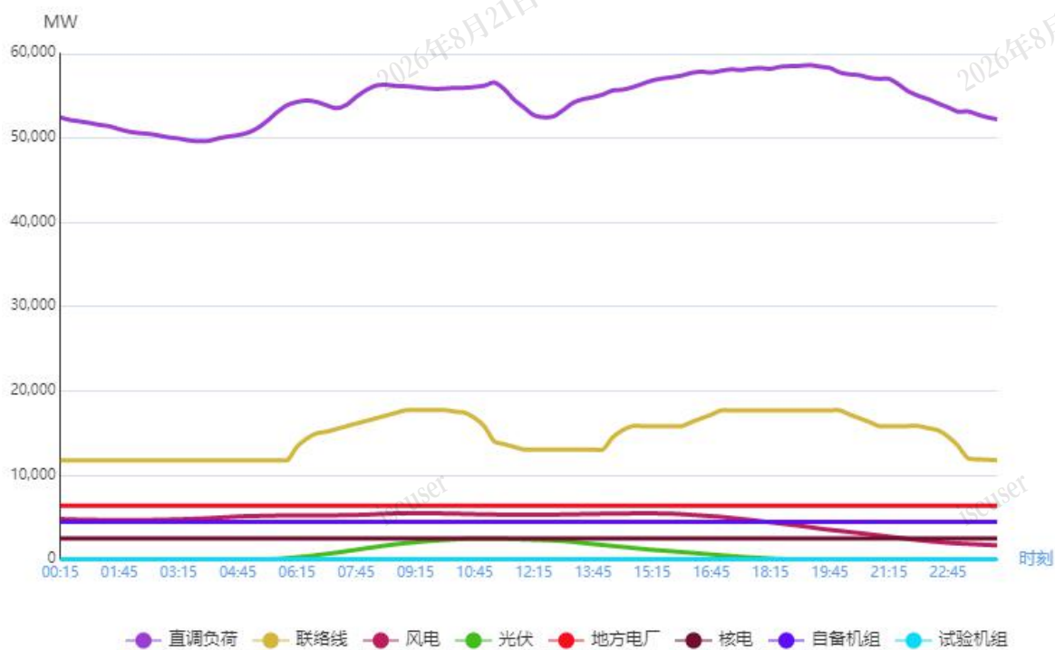
图 2 4 月 28 日负荷及电源出力预测情况
