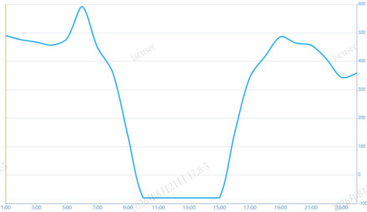
图3 5月2日日前市场用电侧价格
