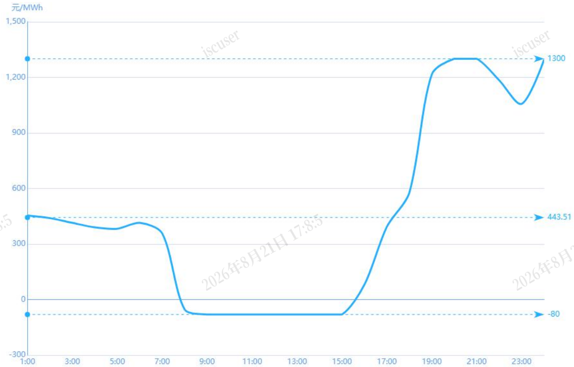
图 4 5 月 1 日实时市场用电侧价格
