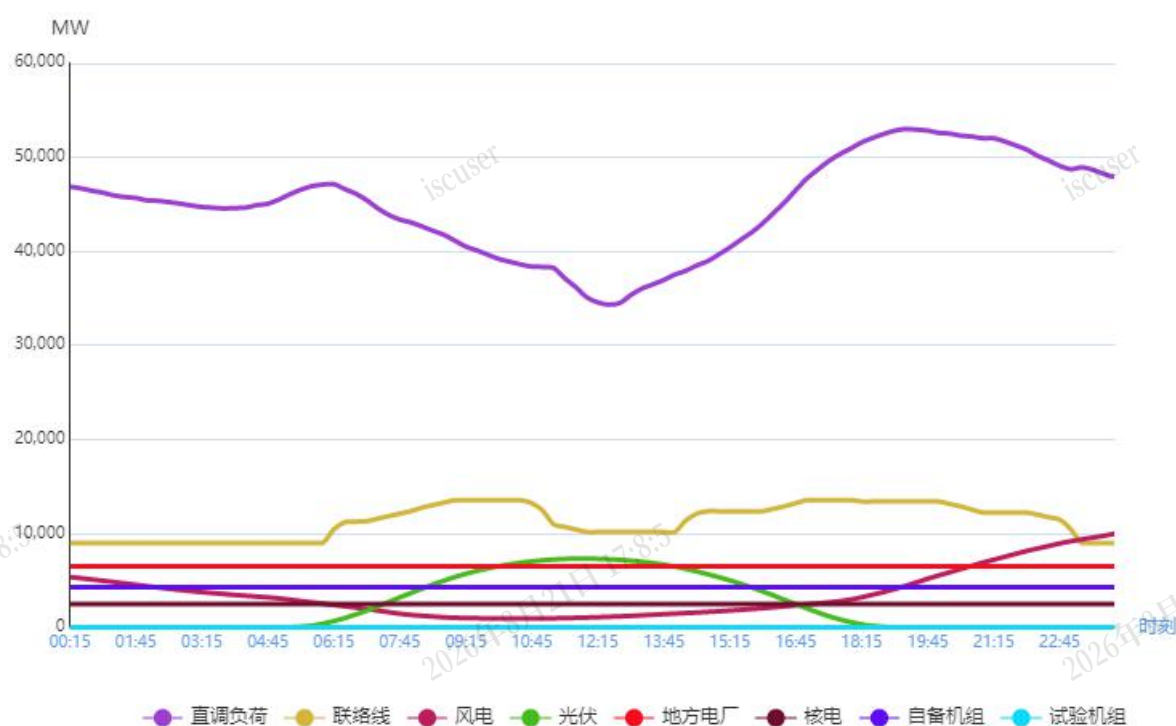
图2 5月2日负荷及电源出力预测情况
