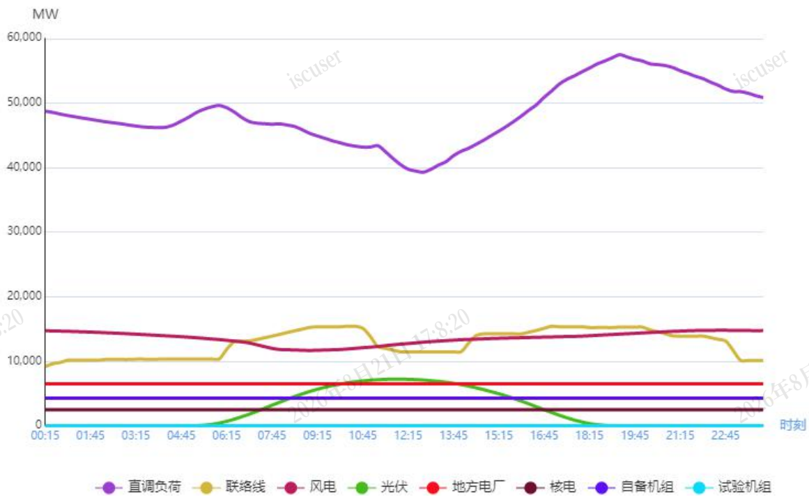
图 2 5月4日负荷及电源出力预测情况
